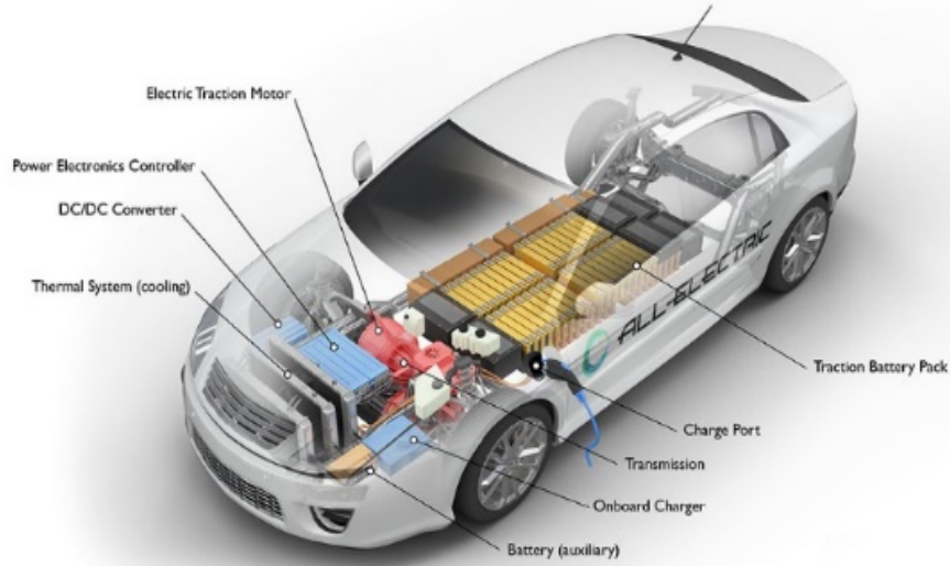
Fig. 6 EV subsystem
